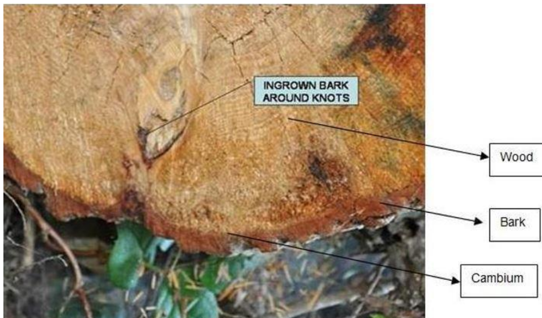
Рисунок 2. Поперечный срез круглого лесоматериала. Рисунок предоставлен С. Села, Канадское агентство по контролю качества пищевых продуктов.
